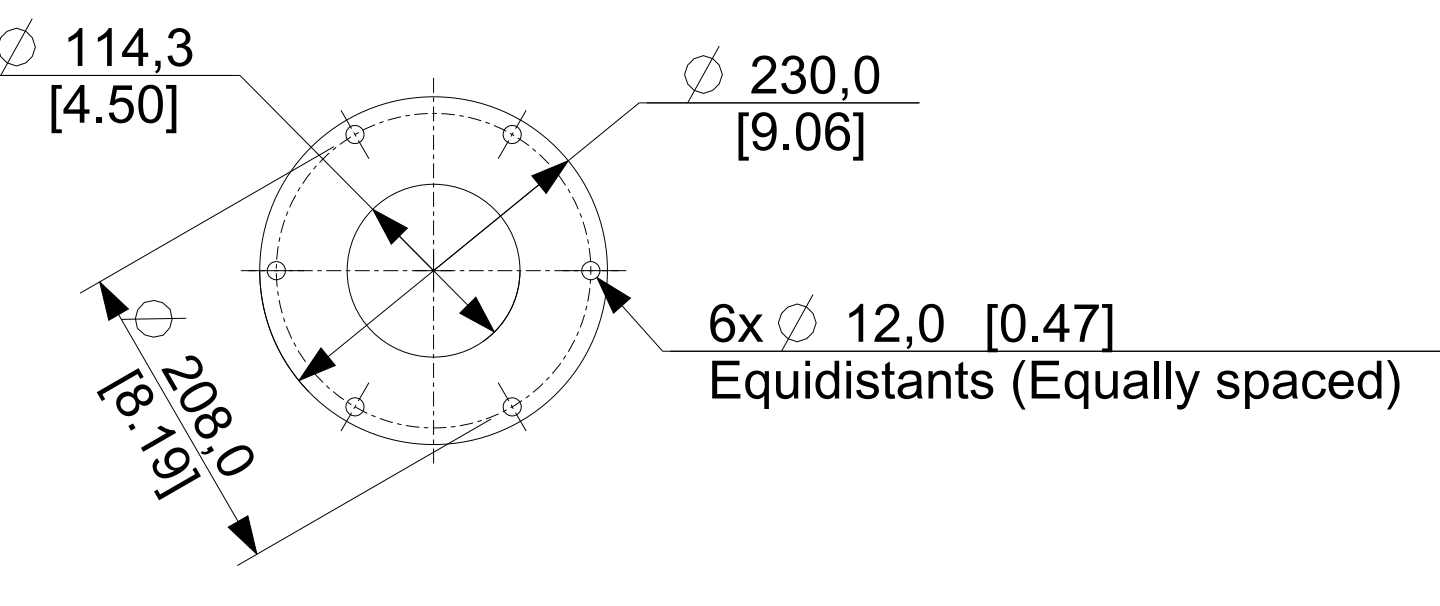
DETAIL : BRIDE SORTIE ECHAPPEMENT MOTEUR / ENGINE EXHAUST OUTLET FLANGE
