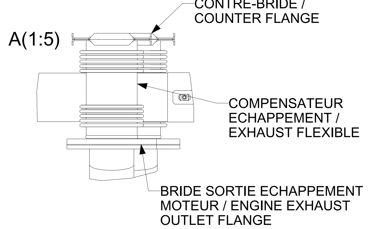
DETAIL : BRIDE SORTIE ECHAPPEMENT MOTEUR / ENGINE EXHAUST OUTLET FLANGE
