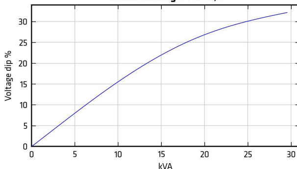
Motor Starting @ P.F. 0,3
